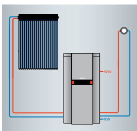
Przykładowy system grzewczy z Vitosolar 300-F i kolektorami Vitosol do podgrzewu c.o. i c.w.u.
